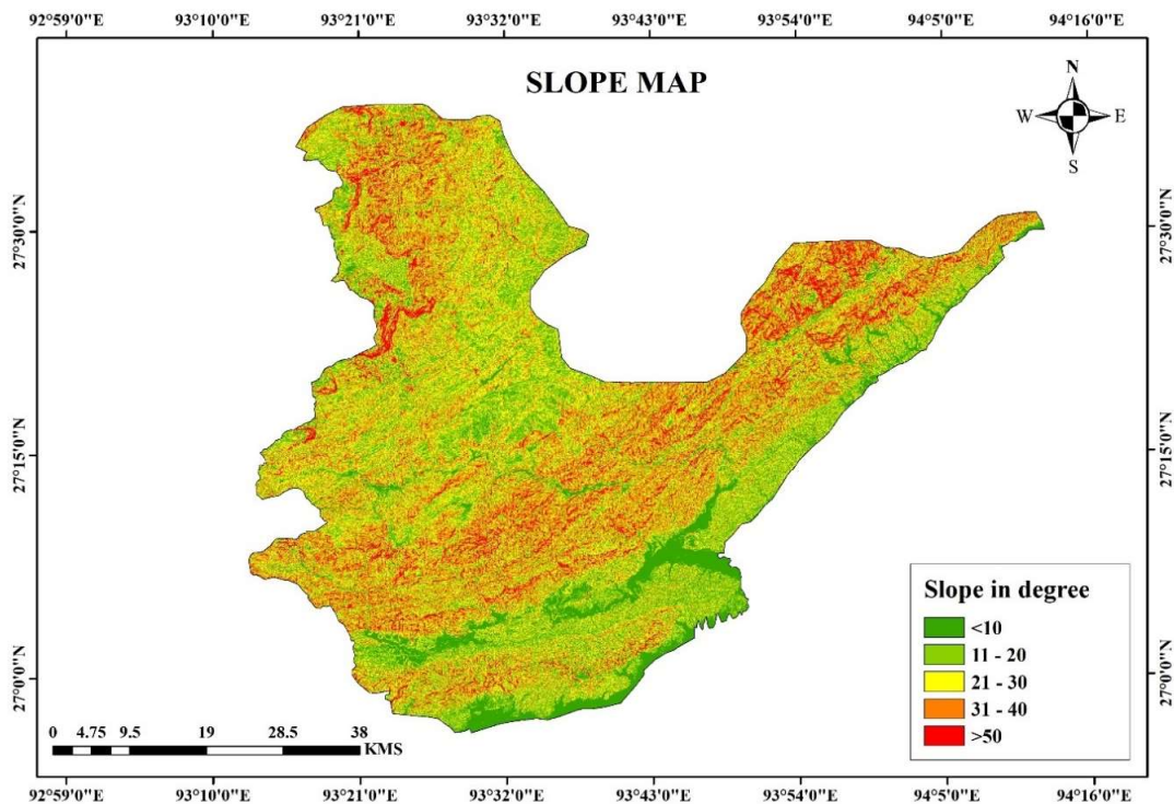
Fig. 3: Slope map.
