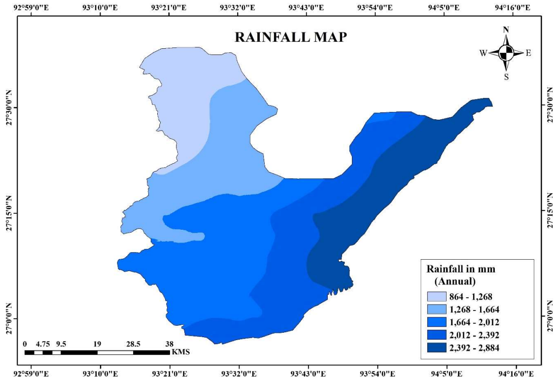
Fig. 4: Rainfall map.
